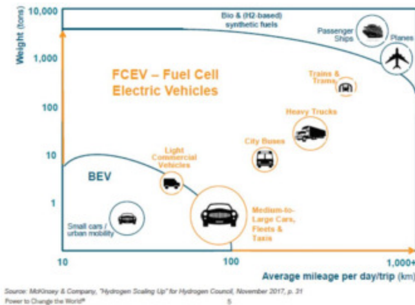
Abbildung 2: Einsatz verschiedener Antriebsarten nach Reichweite und Gewicht. (Kreitmaier 2019:3)
